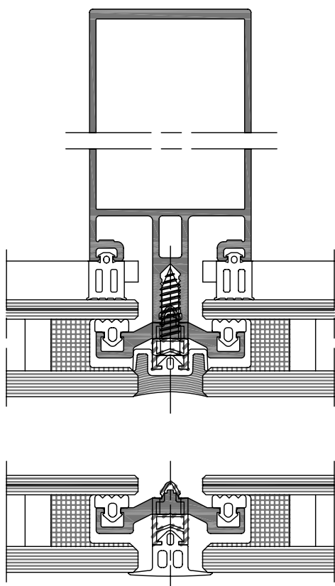
Sezione orizzontale
